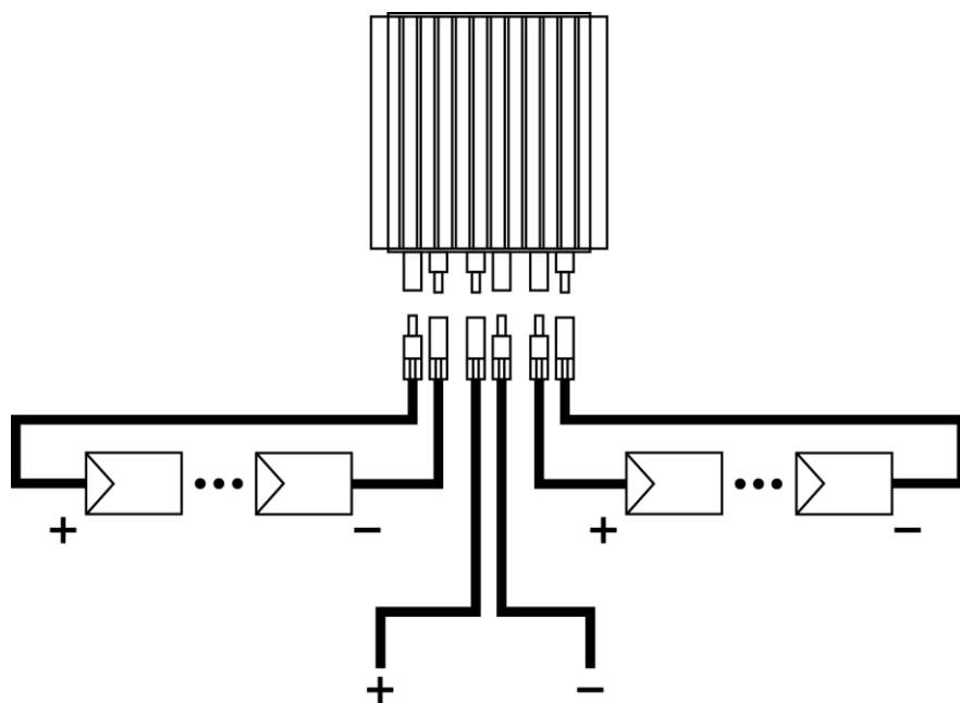
図 7: ストリングオプティマイザの出力回路用の差込形接続端子のオス／メスと極性
