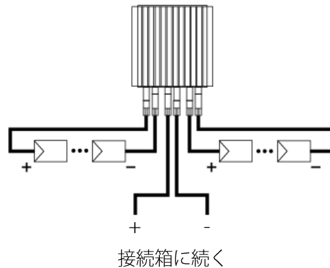
図 13: コネクターがしっかり閉まっていることを確認
