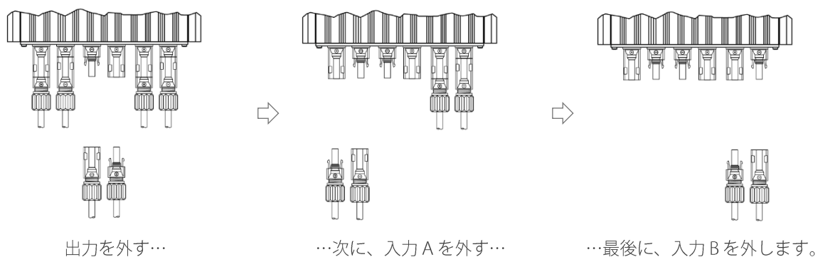
図 19: 外す順序が重要です
