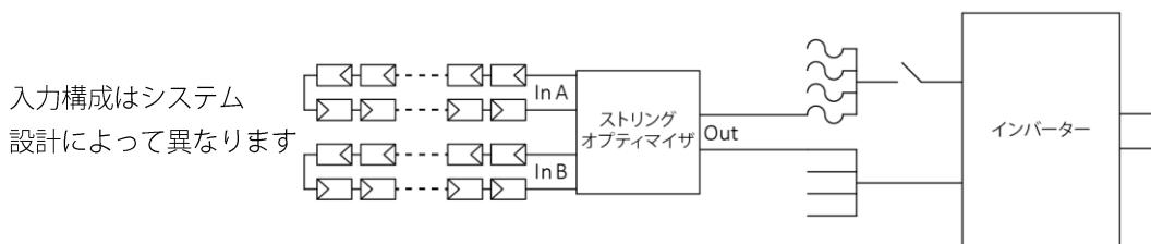
図5: 接地 PV アレイの電気接続
