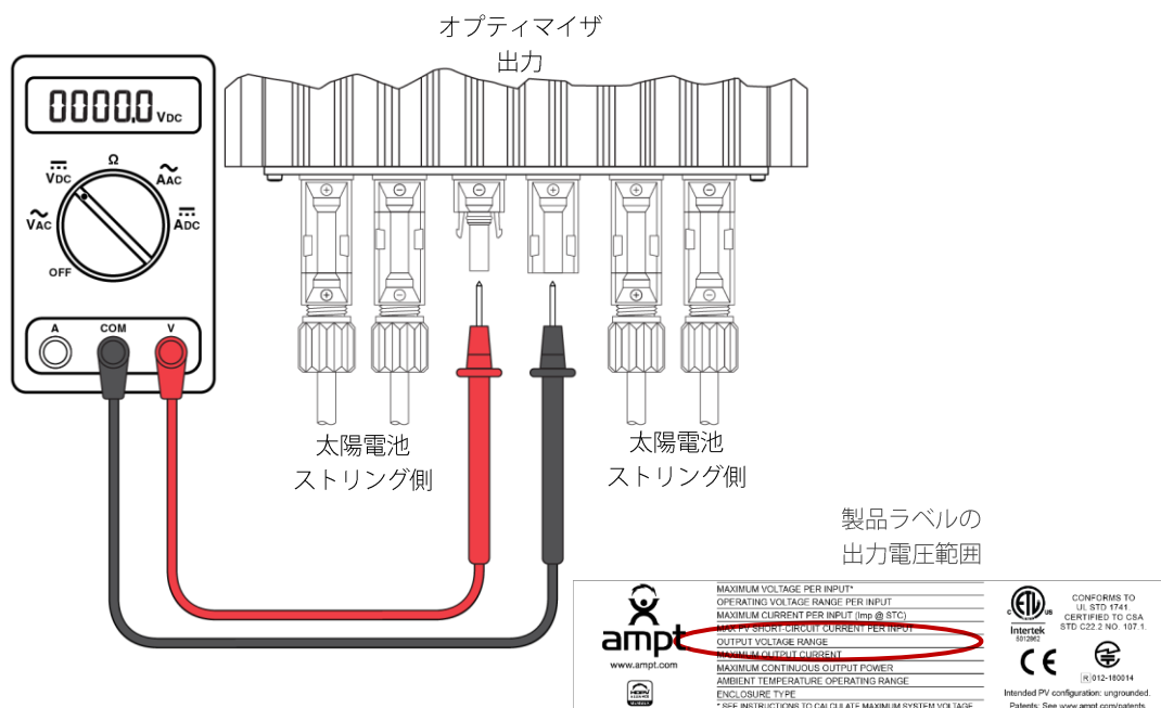
図 15: 適切に設置されているか確認
