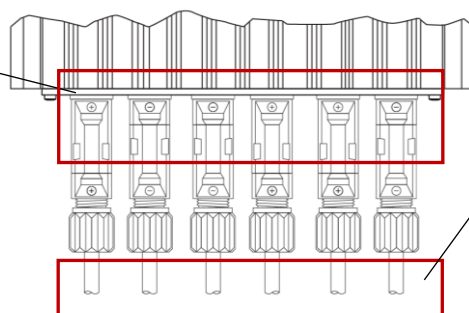
図 17: コネクタが完全にはめ込まれていることを確認し、コネクタに張力がかからないようにケーブルを整線します
