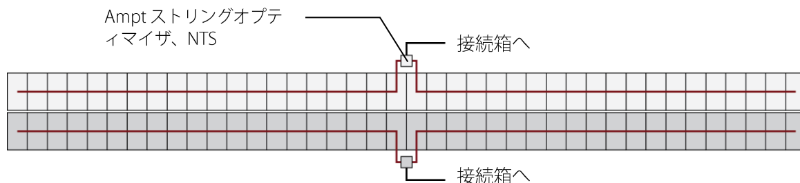
図 9: アレイ間に陰が生じる場合の配線例
