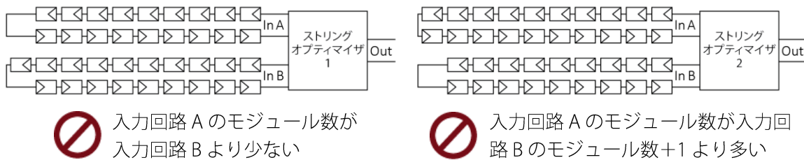
図7: 不可能な入力回路構成
