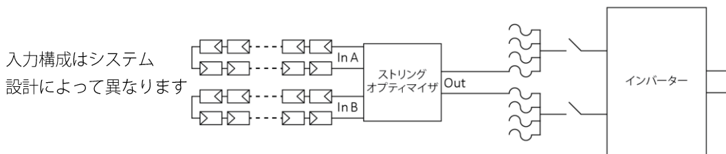
図4: 非接地 PV アレイの電気接続
