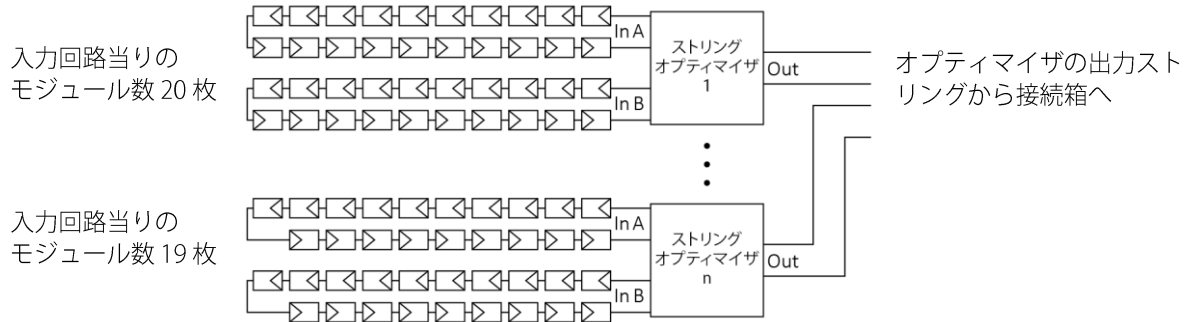
図8: 並列するオプティマイザ間の各入力回路に接続するモジュール数は、可能な入力配列基準を満たし、Ampt の設計ガイドラインに従う限り、変則的に設定できます。
