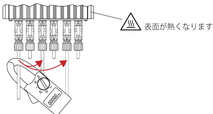
図 18: オプティマイザ回路に電流が流れていないことを確認します
