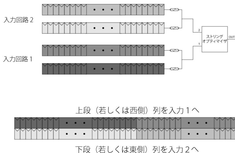
図 9: 発電量を最大化するために、同じ列のモジュールは同じ 옵ティマイザ入力に接続してください。
