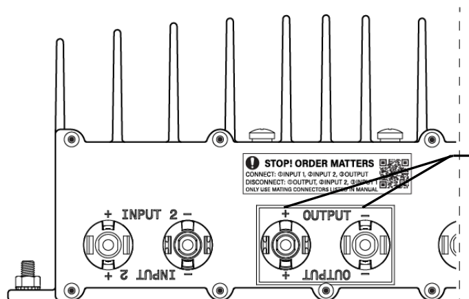
オプティマイザ 正面図
