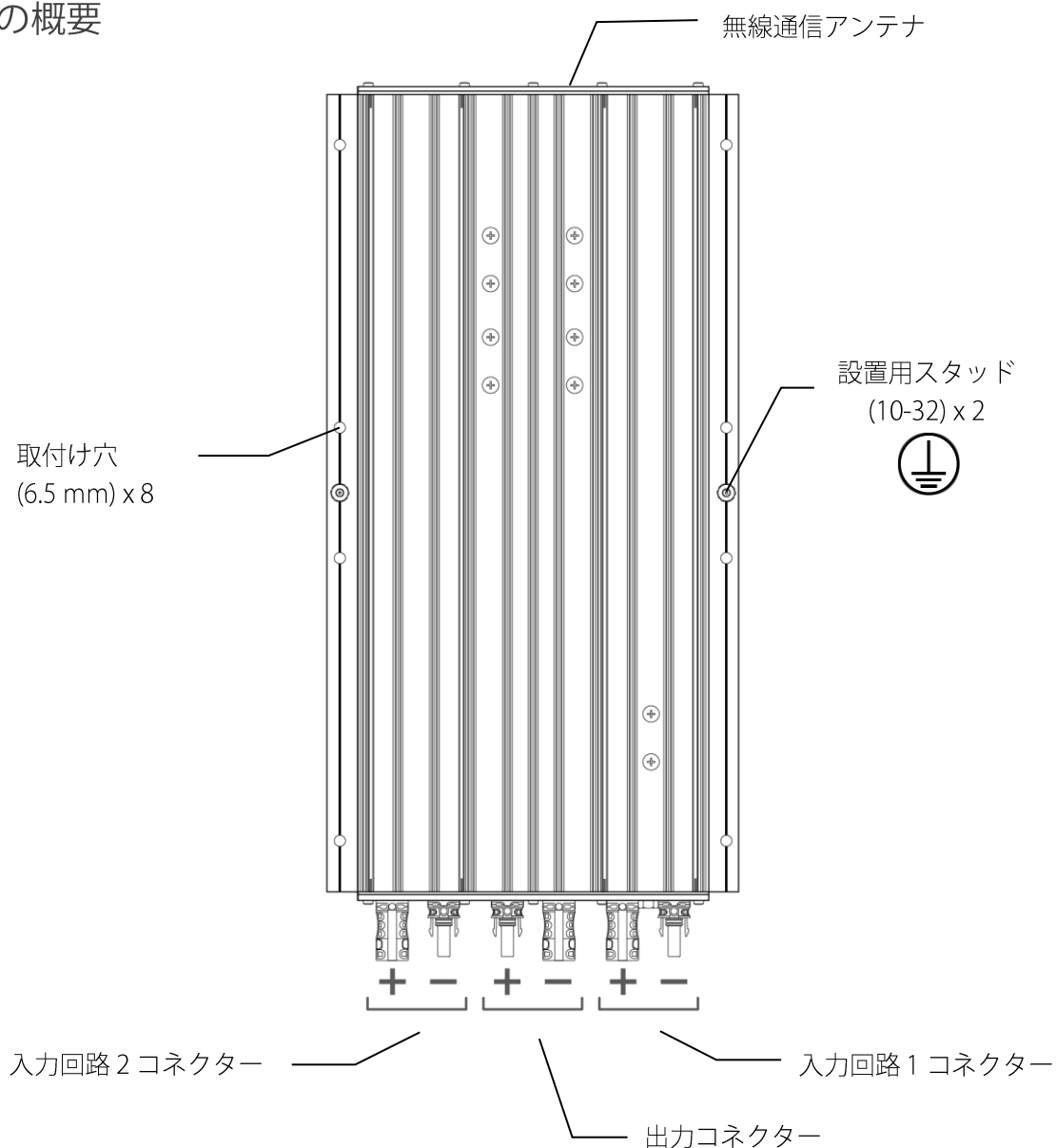
図 2: Ampt スtring オプティマイザの各部の概要
