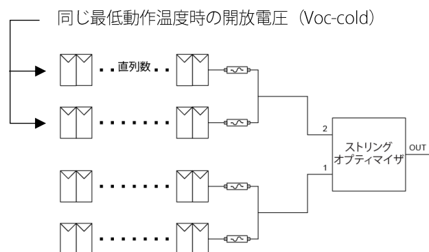
図 6: 例—2 スtring スを並列して各入力回路に接続
