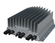
i13.5ストリングオプティマイザ システム電圧: 600 – 1000 V 出力電流: 12 – 13.5 A 出力電力: 5.9 – 12.2 kW
